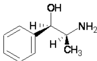
(1 R ,2 S )-2-amino-1-phenylpropan-1-ol
